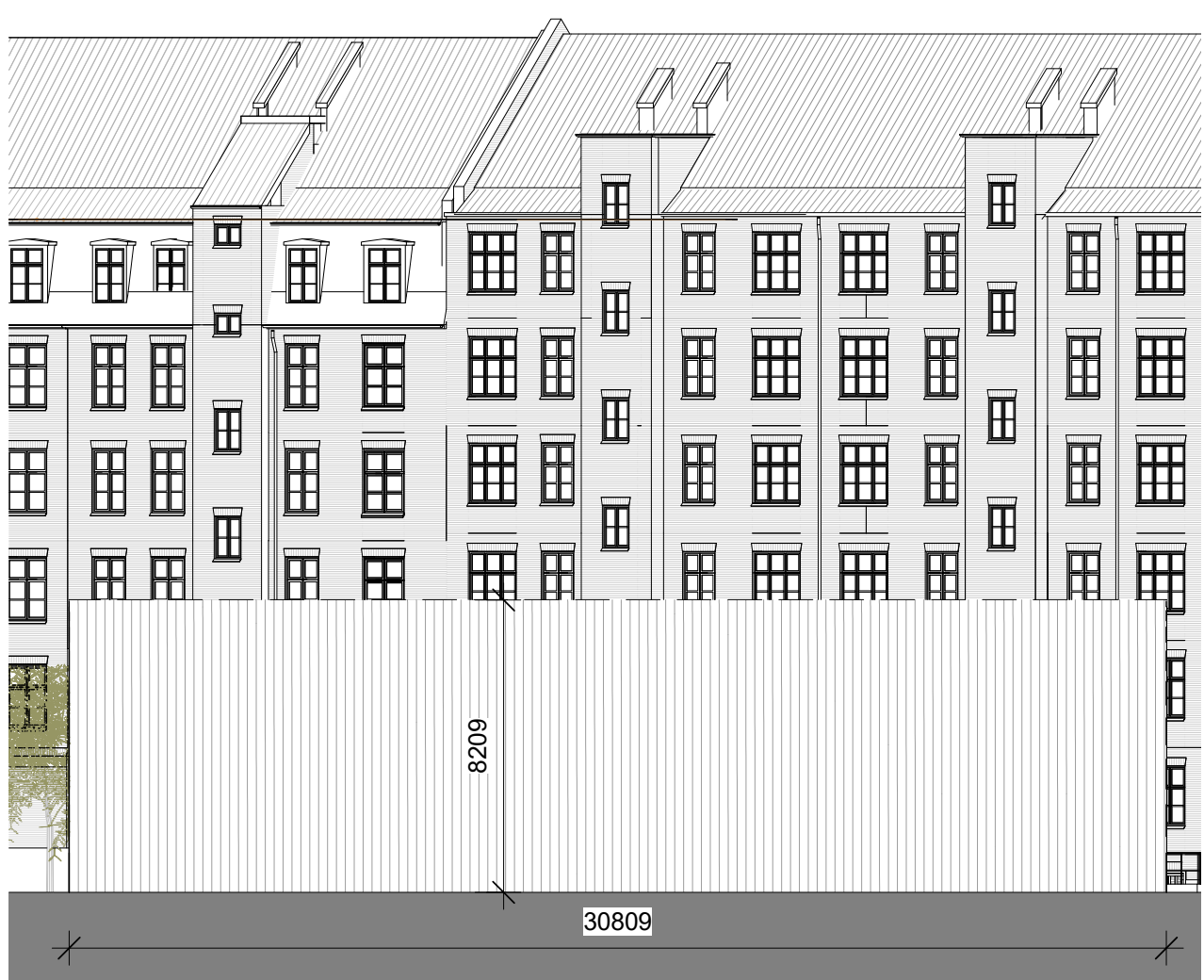
Syd facade 1 : 200
